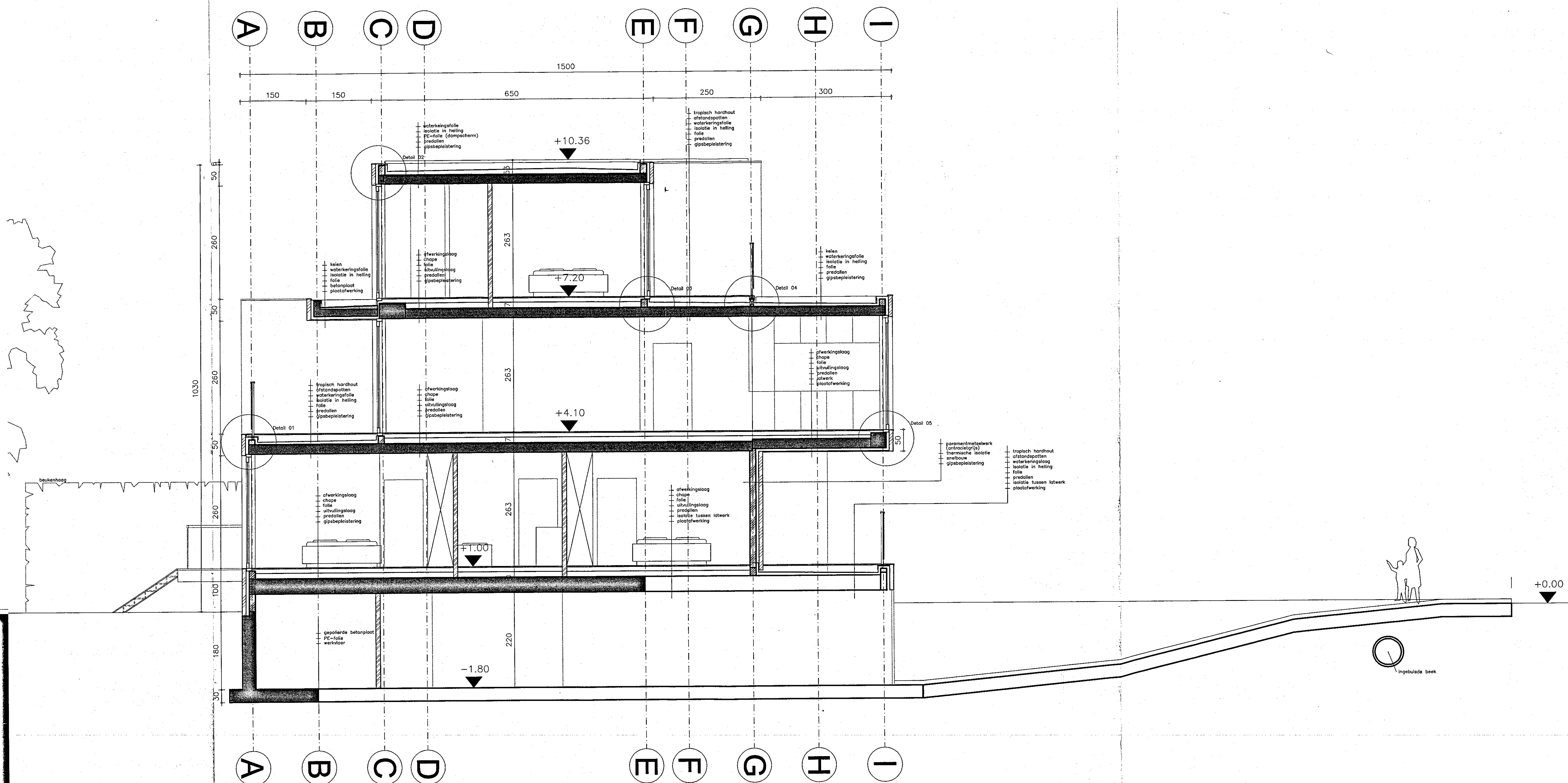
LANGSSNEDE DD' 1/50
