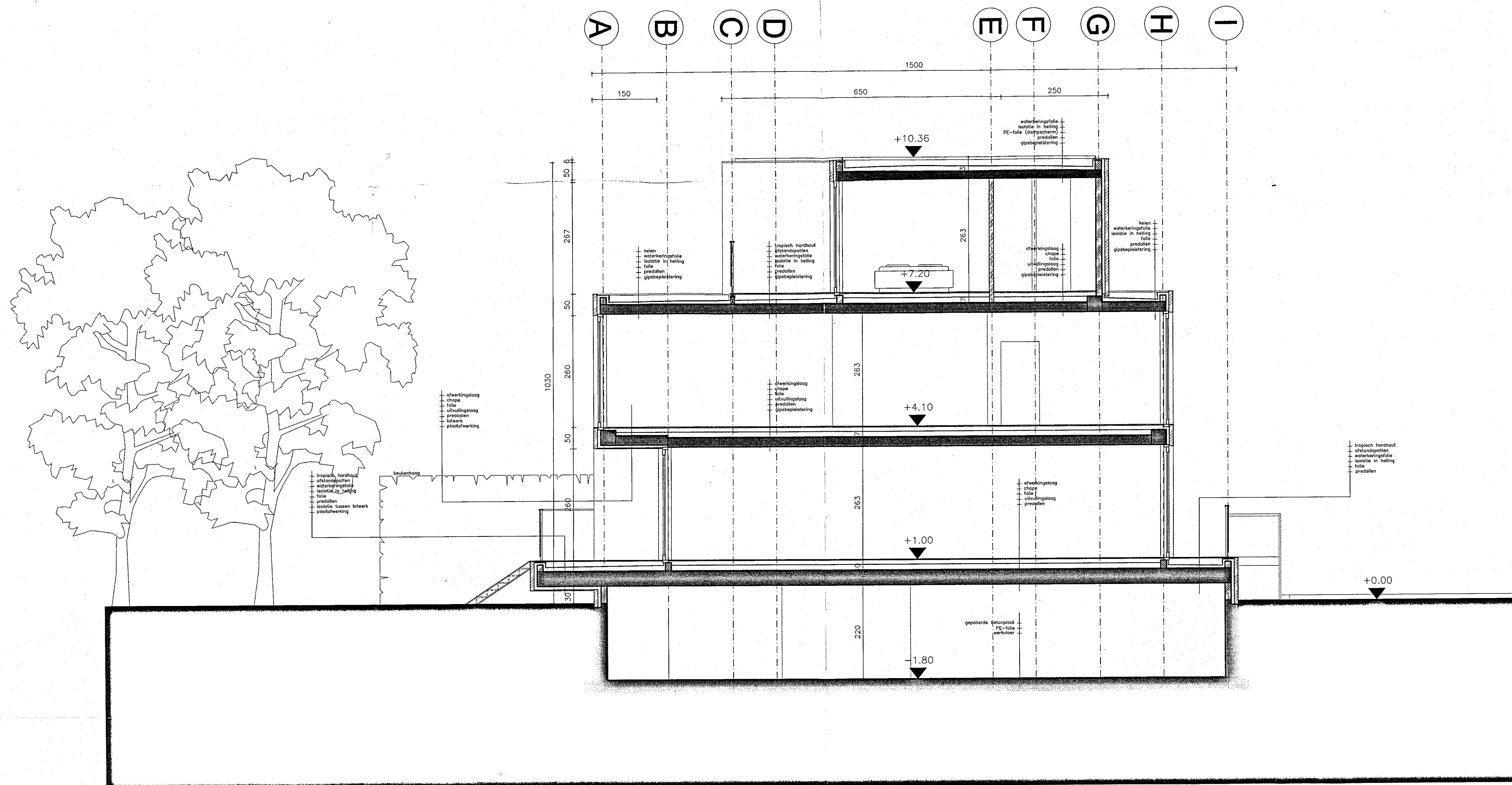
LANGSSNEDE CC' 1/50
