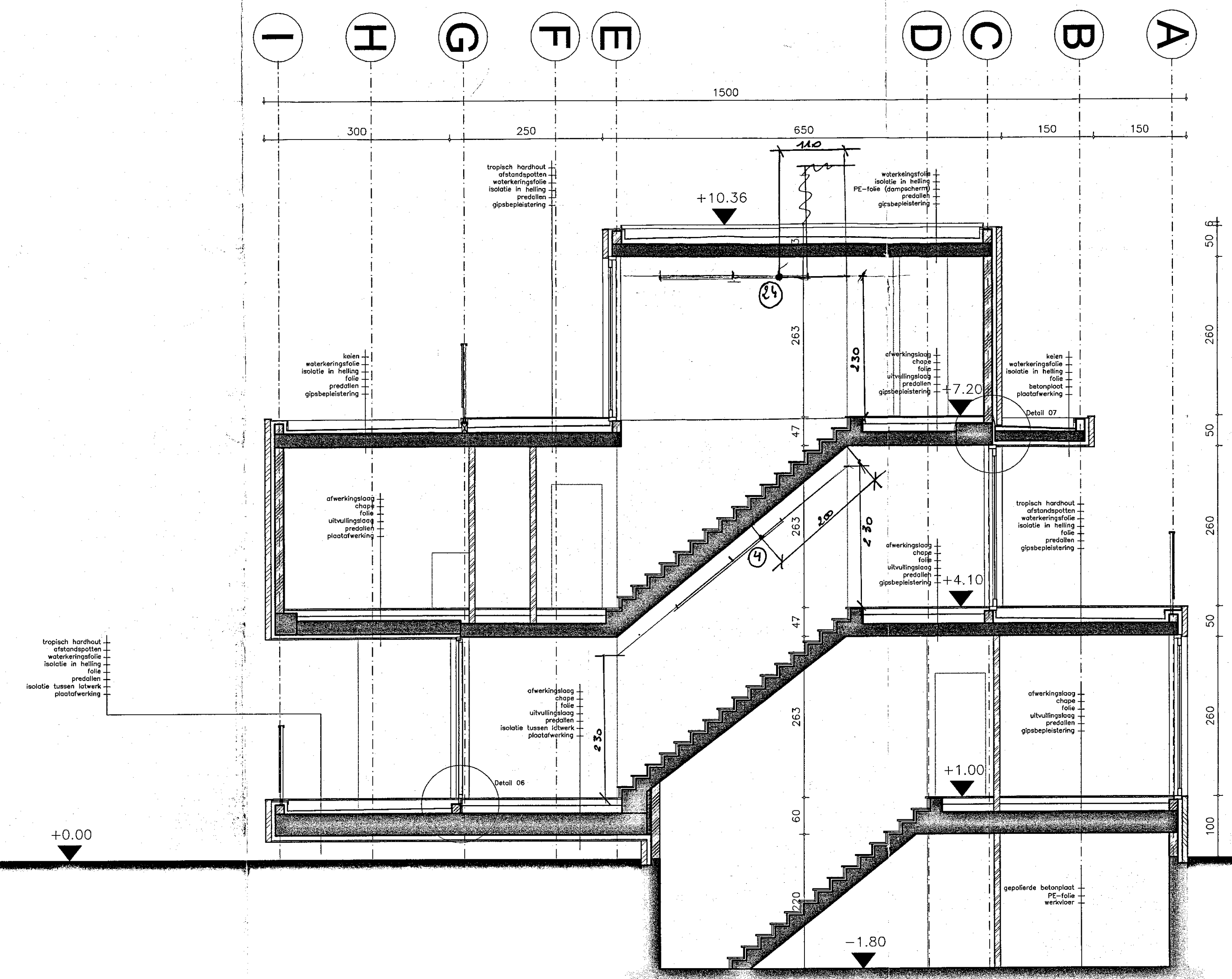
LANGSSNEDE BB' 1/50
