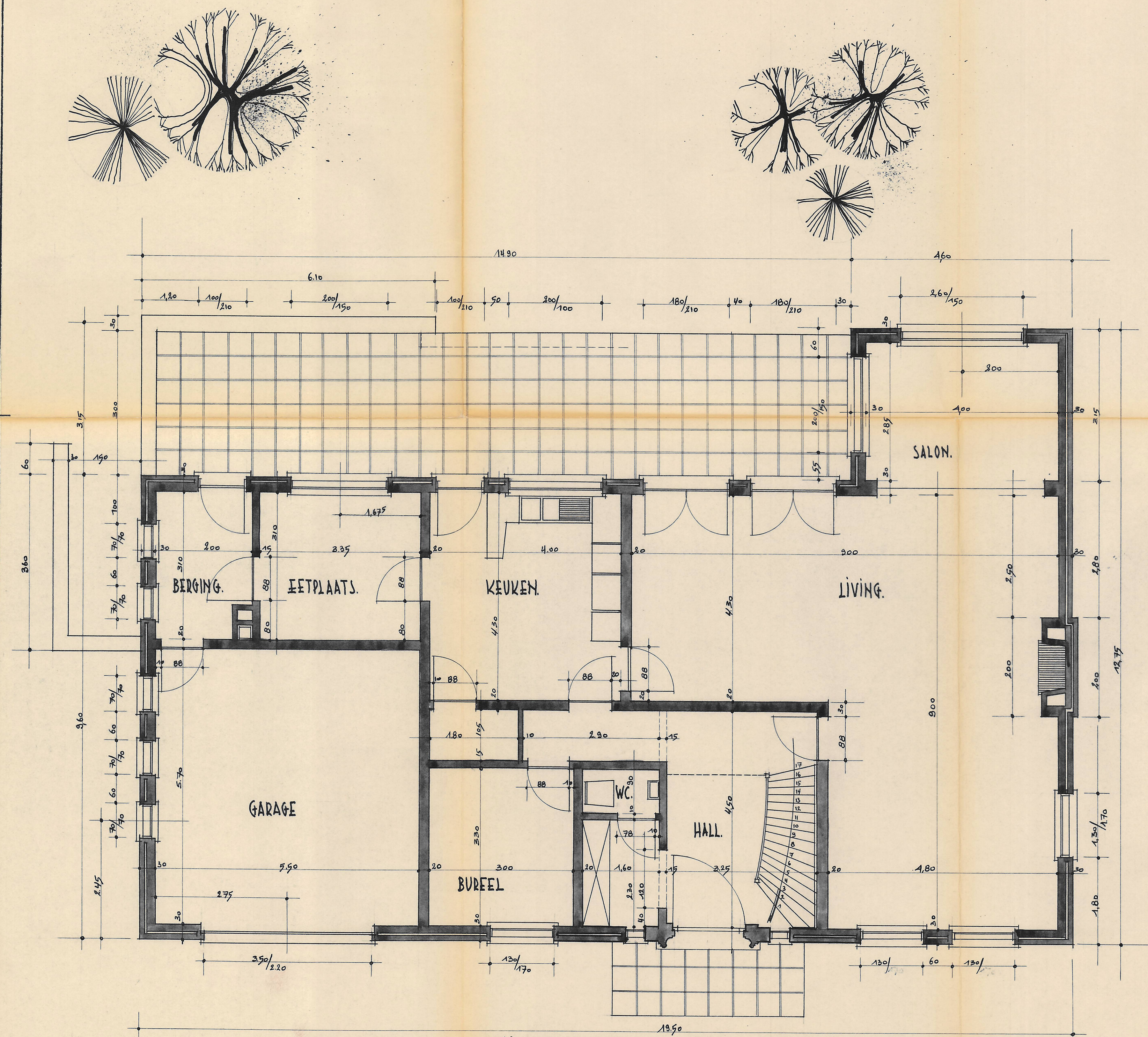
PLAN GELIJKVLOERS
