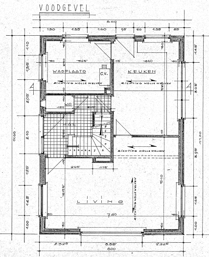
PLAN GELUKVLOERS 2:100
