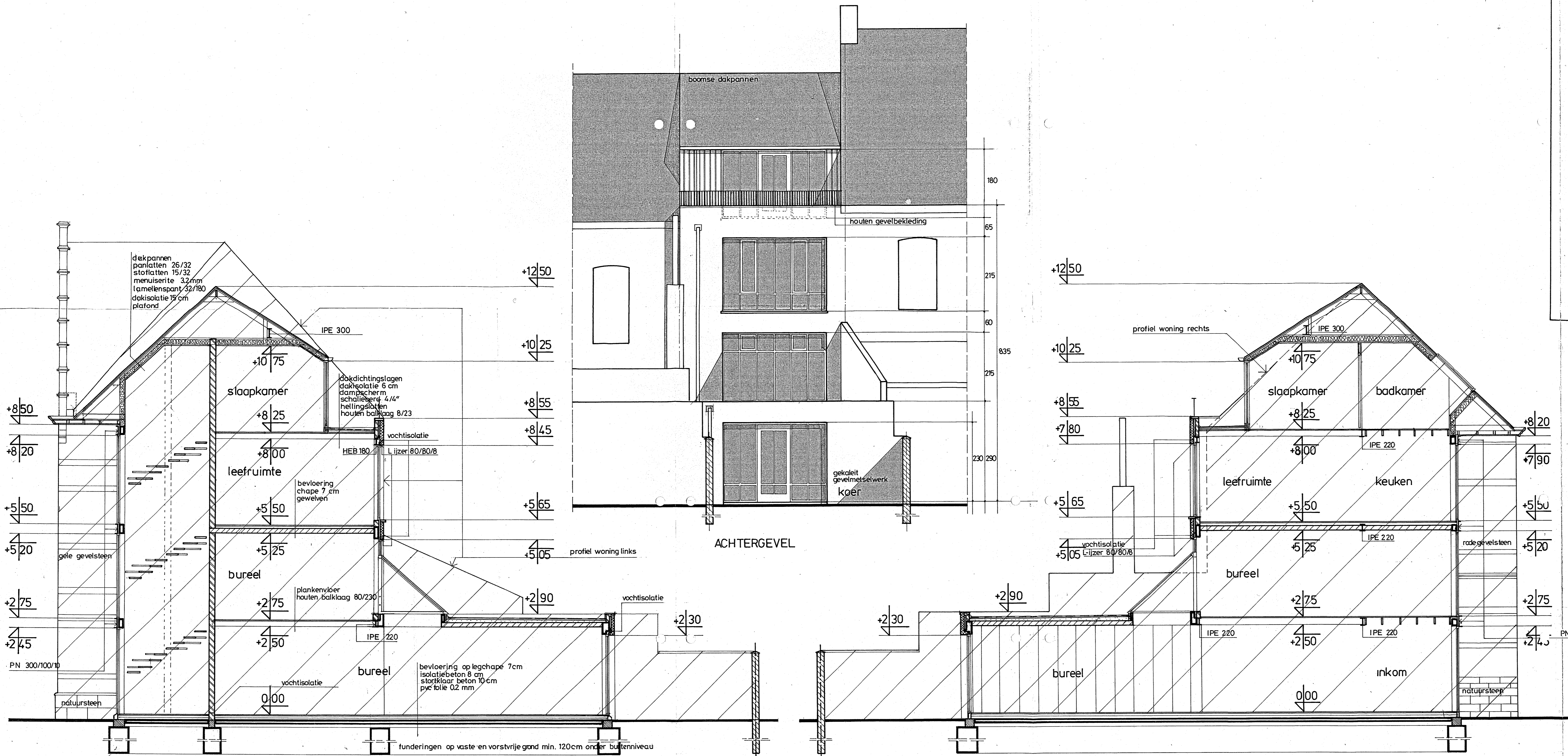
DOORSNEDE A-A
