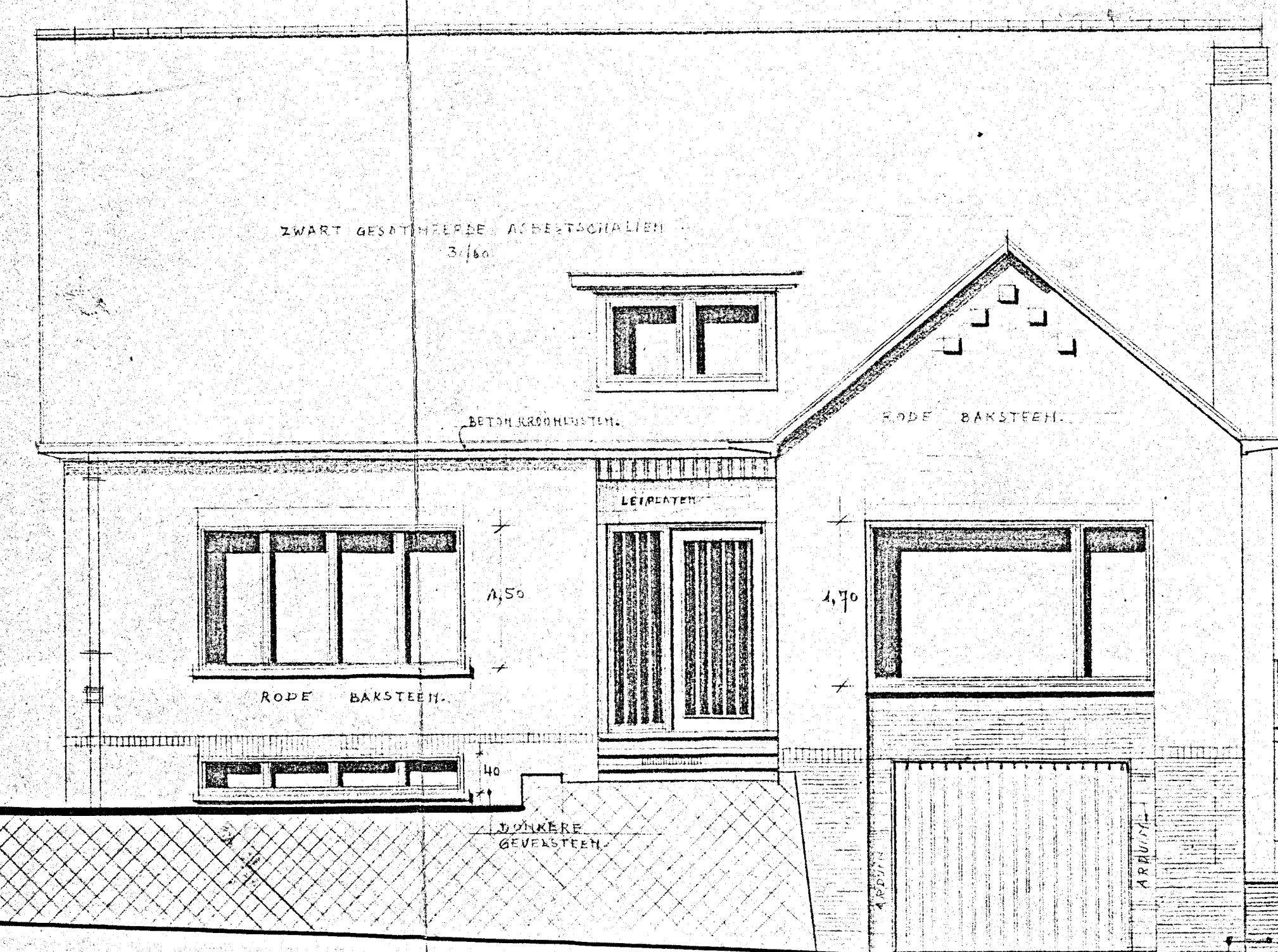
VOORGEVEL.
