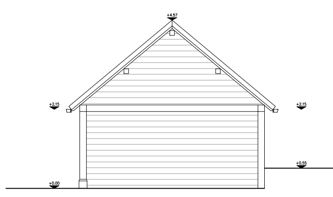
RECHTER ZIJGEVEL
