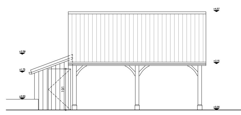
VOORGEVEL
