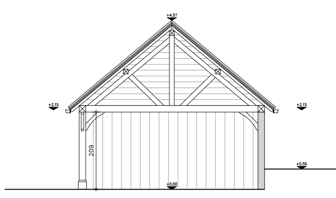
SNEDE AA'
