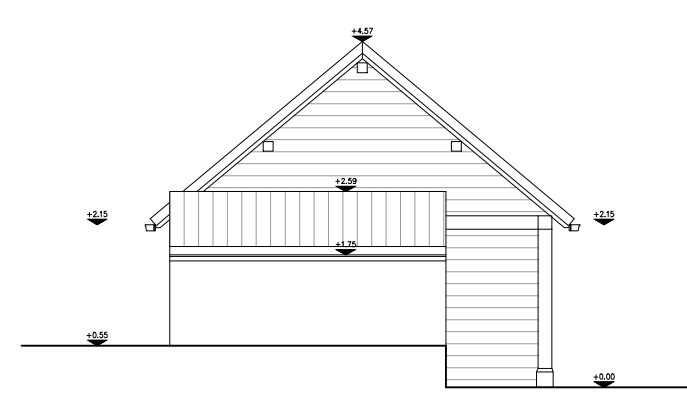
LINKER ZIJGEVEL
