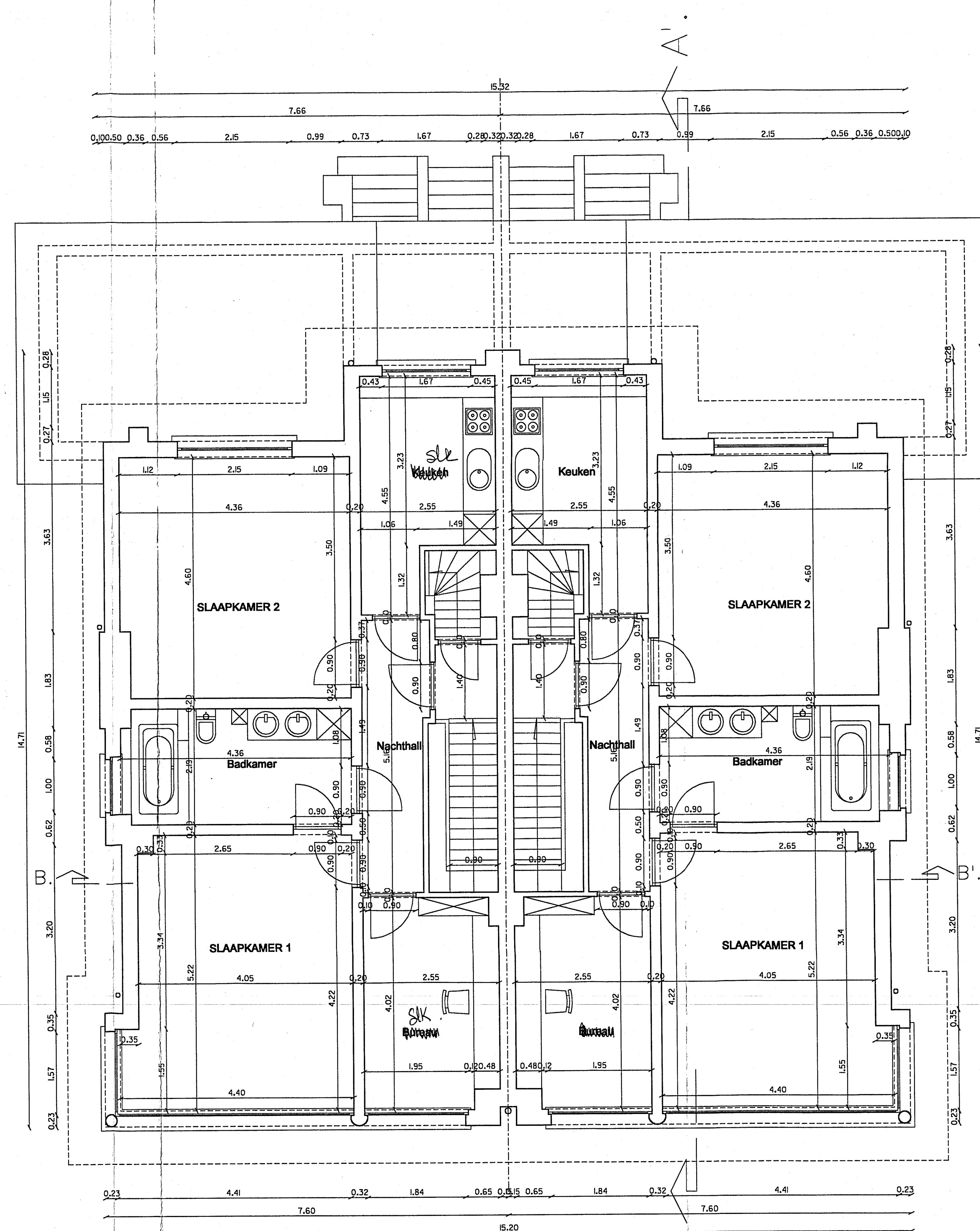
Verdiepingsplan
