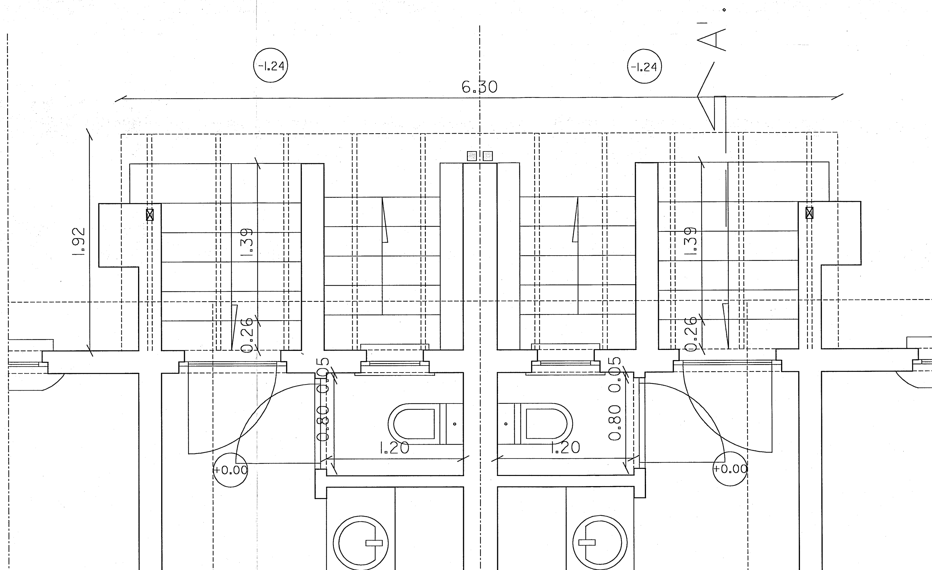
Gelijkvloers 1/20
