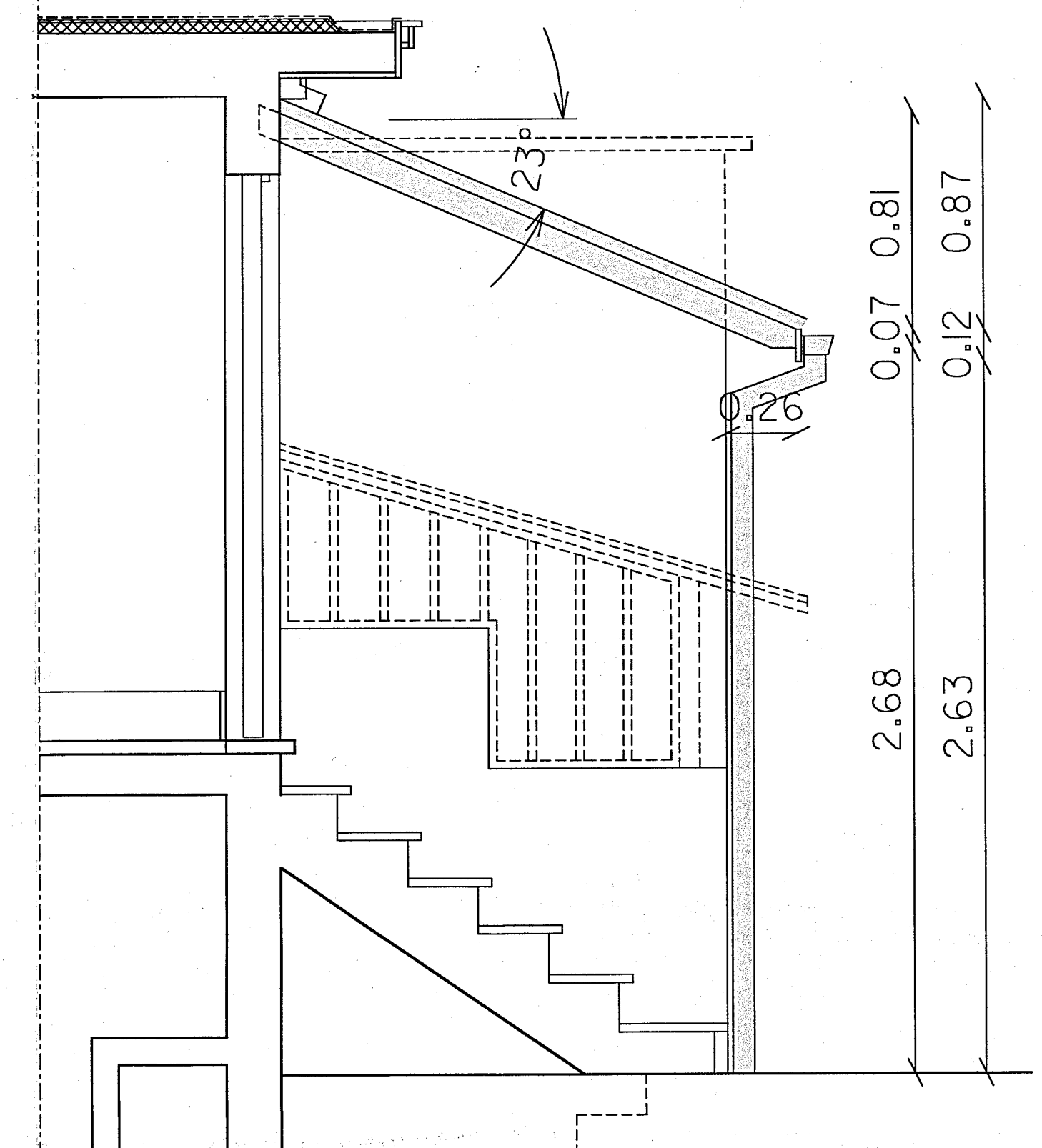
Sede A-A' 1/20
