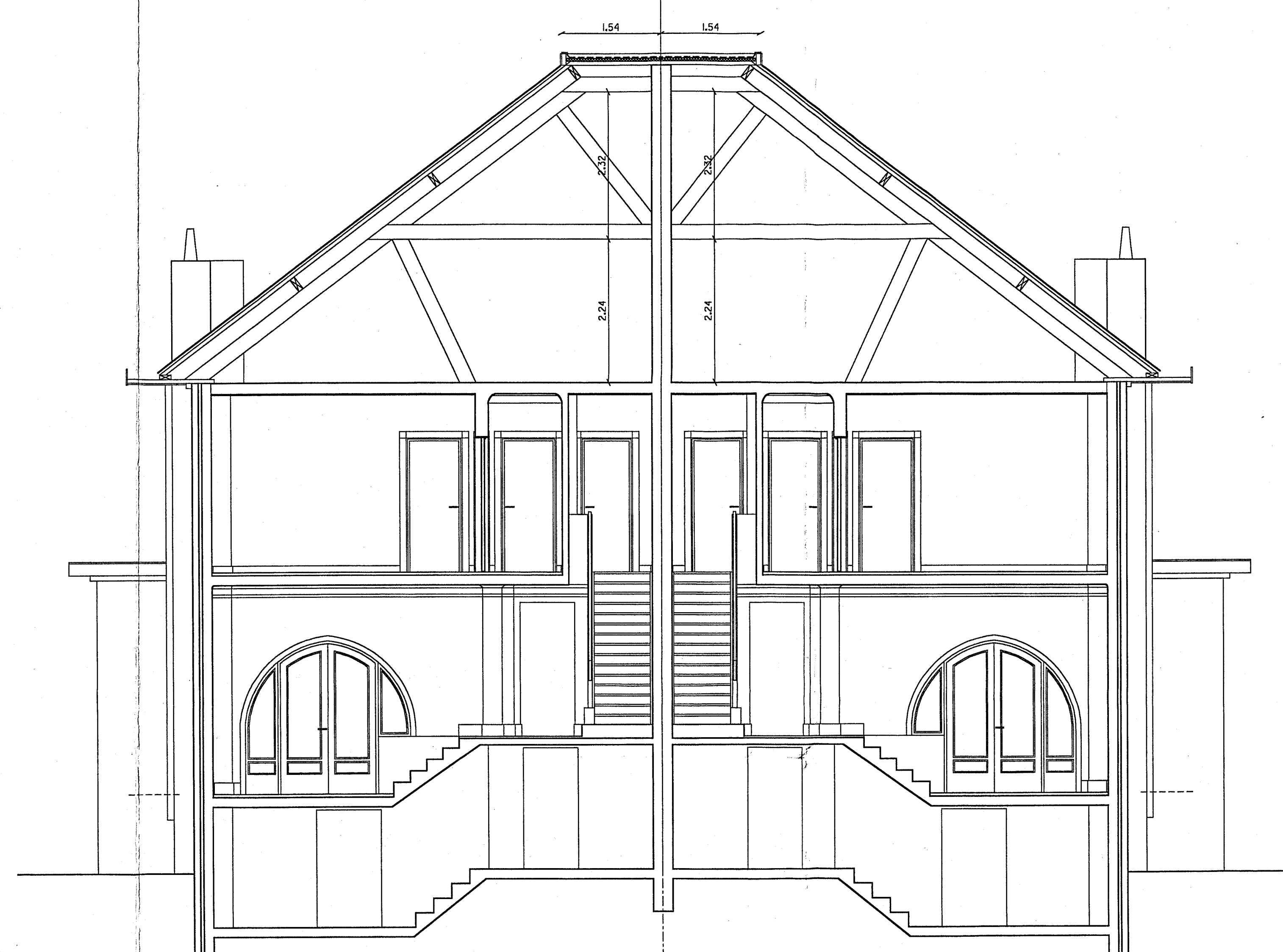
Snede B-B'
