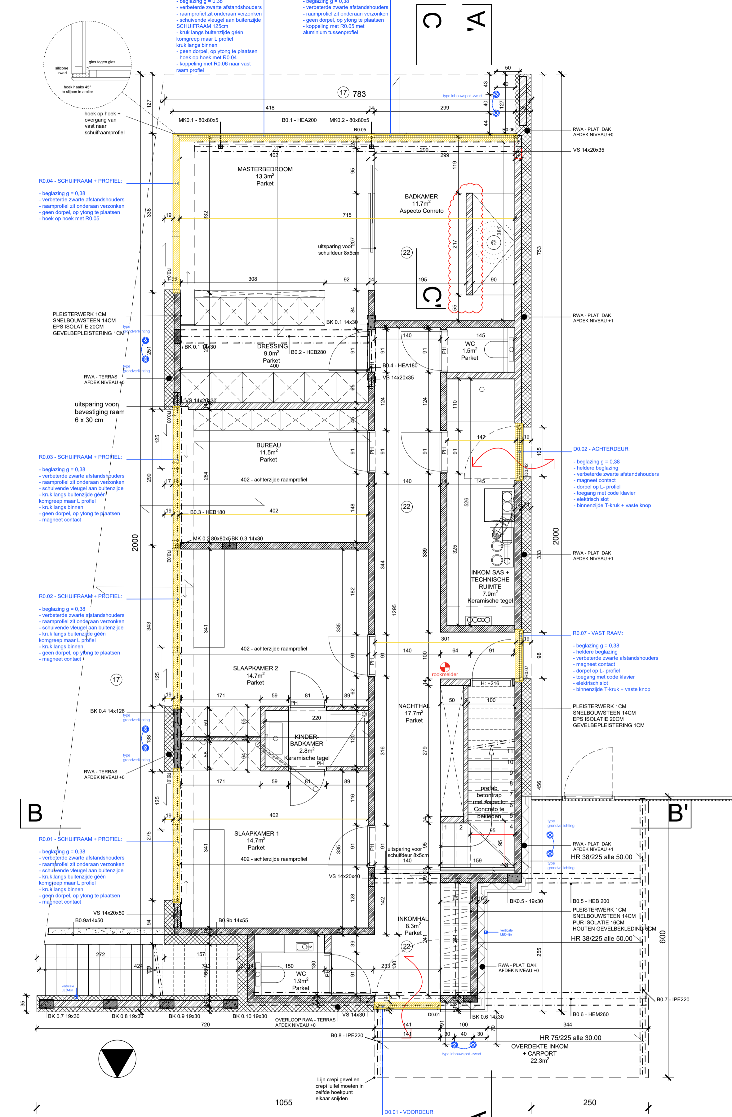
PLAN NIVEAU 0 WONING - BRUTO OPP: 139.8m 2 - excl. tuinmuur, buitentrap en luifel (opp luifel: 35.4m 2 )
