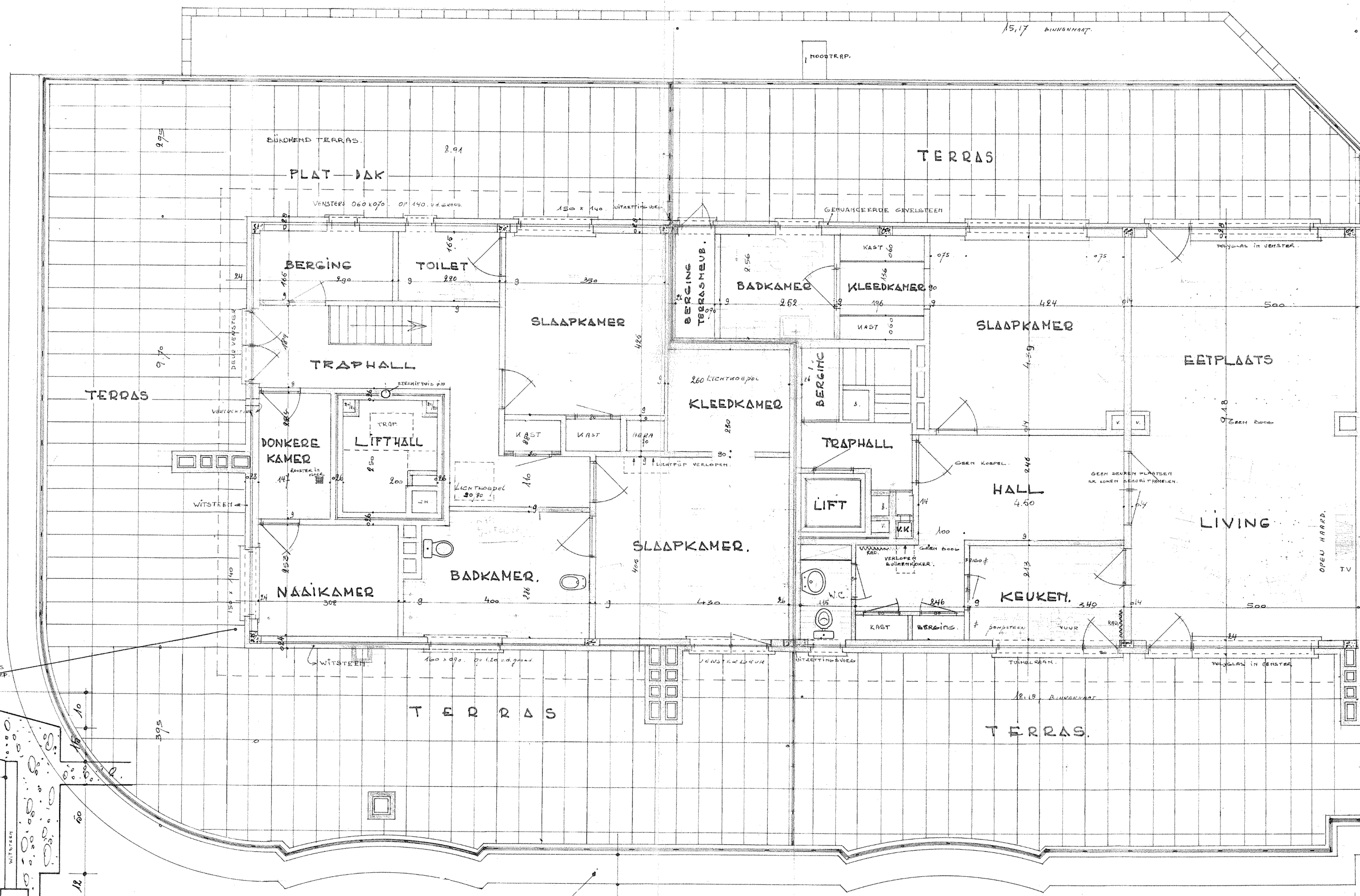
PLAN APPARTEMENT 9 B.
