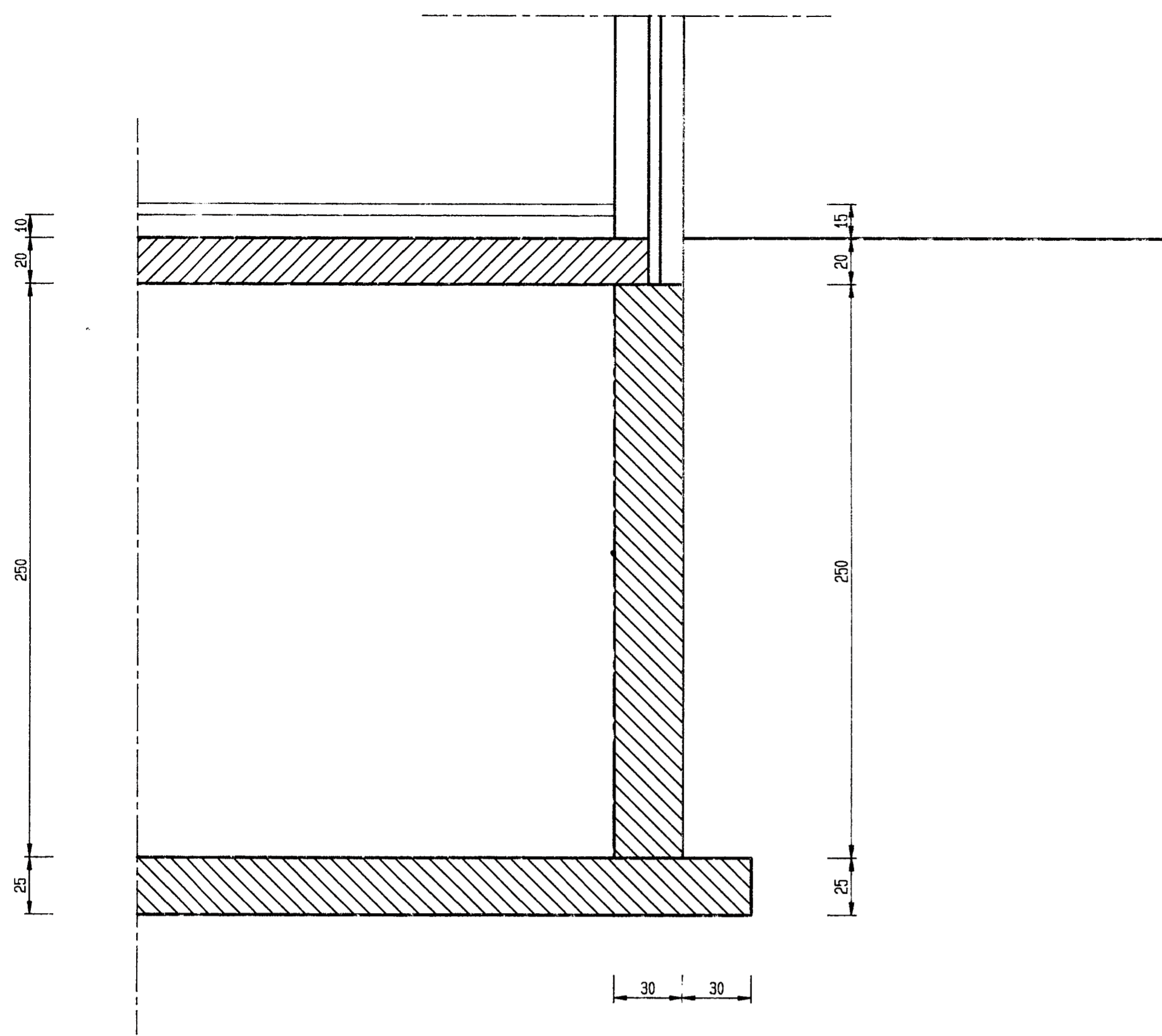
DOORSNEDE (schaal 5 %)
