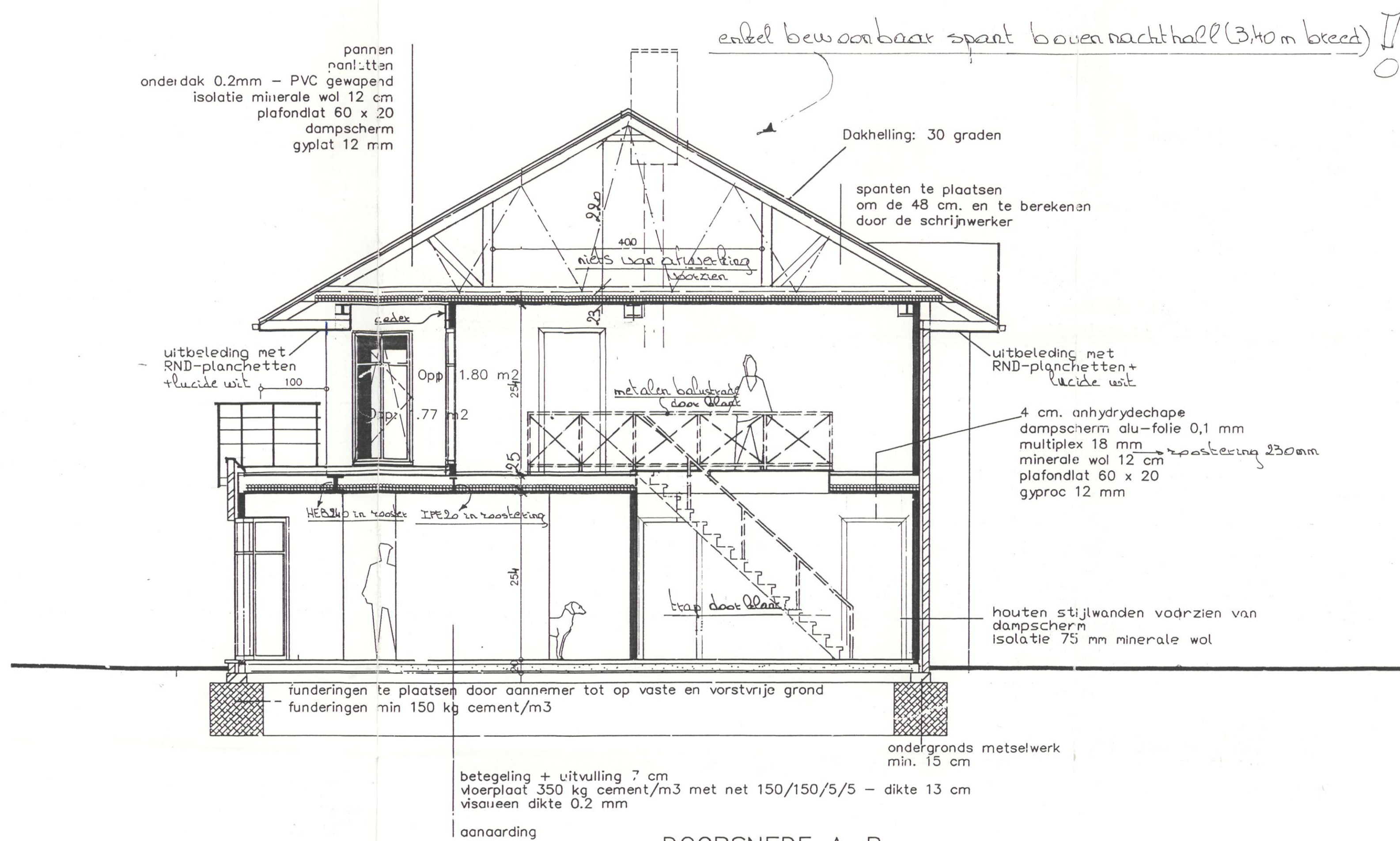
DOORSNEDE A-B
