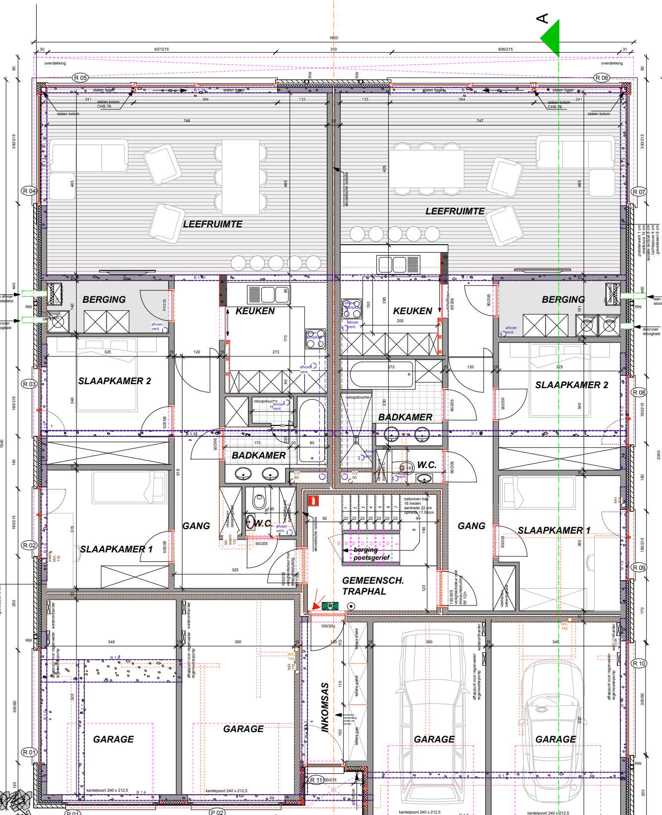
PLAN GELIJKVLOERS SCHAAL 1/50
