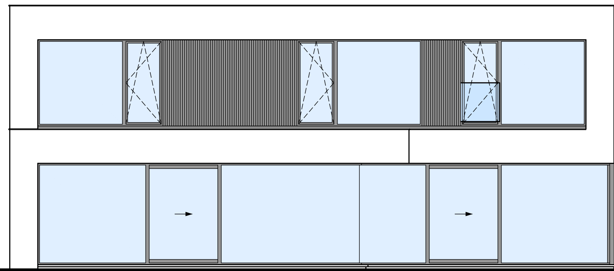
Achtergevel schaal 1/50
